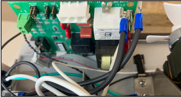
11. Instale la nueva tarjeta electrónica de reemplazo en la ranura de la placa.
