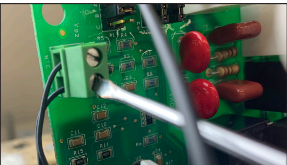
15. Instale los 2 cables en las terminales y utilice el desarmador pequeño plano para apretar los tornillos.
