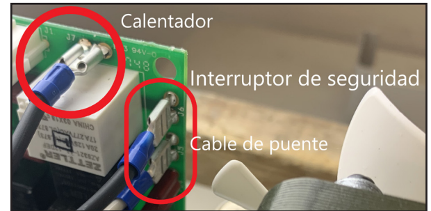
14. Reconecte los (3) cables usando como guía la fotografía que tomo anteriormente (paso #4). En este caso, el cable del calentador va en la parte superior y el interruptor de seguridad cable negro asia el lado de arriba y el cable de puente blanco va abajo.
