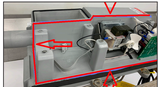
16. Usando el sellador provisto, aplique el sellador a lo largo de la ranura de la cubierta EEC y el módulo central como se ilustra arriba.
