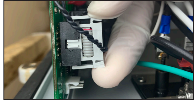
12. Conecte la cinta electrónica del adaptador interfaz.
